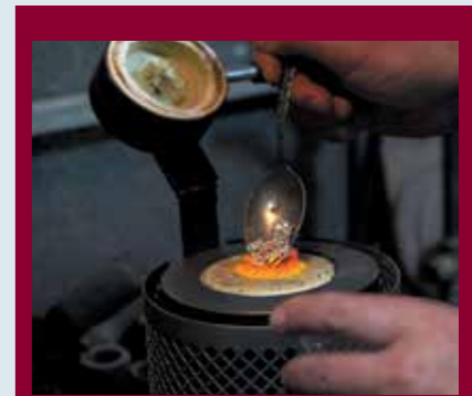
3. Загрузка гранул серебра и легирующих добавок в плавильную печь
